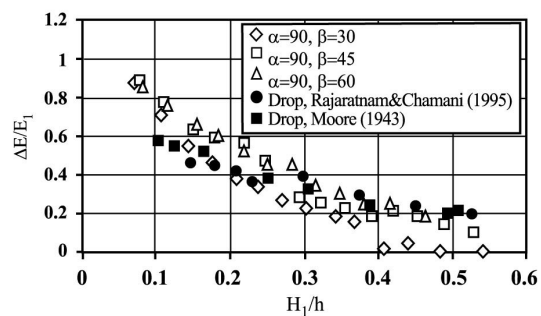
شکل ۱۱- تاثیر تغییرات شیب بالادست سرریز بر افت نسبی انرژی.
