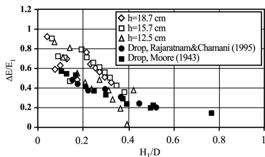
شکل ۱۰- تاثیر تغییرات ارتفاع سرریز بر افت نسبی انرژی.
