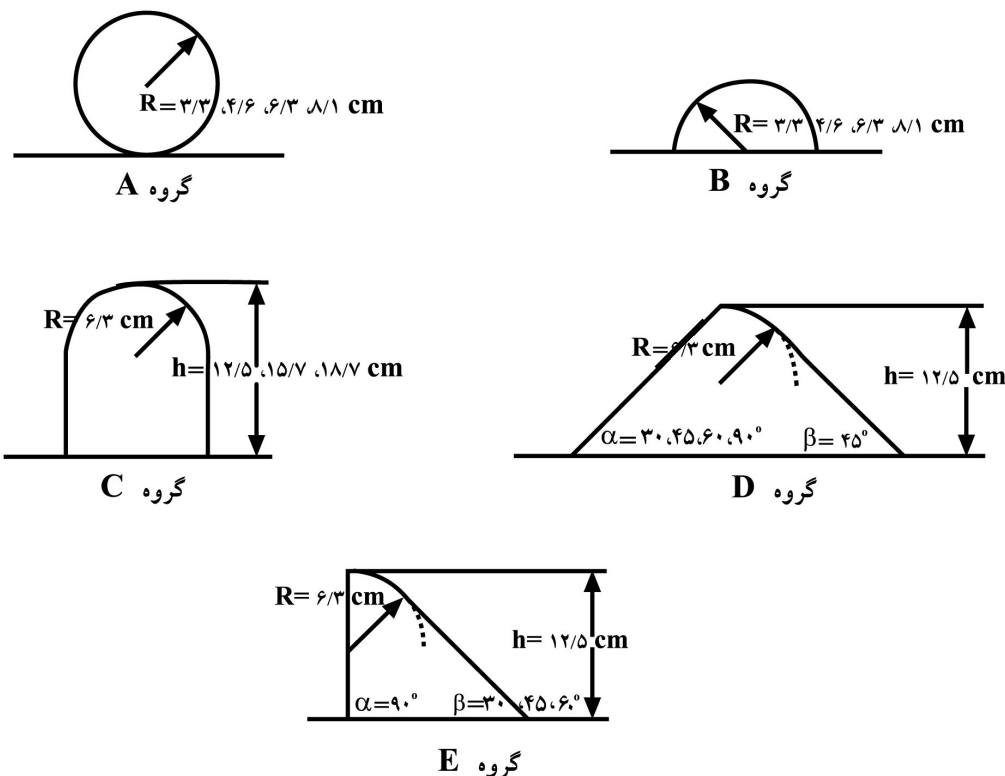
شکل ۲- مشخصات مدل‌های فیزیکی مورد آزمایش
